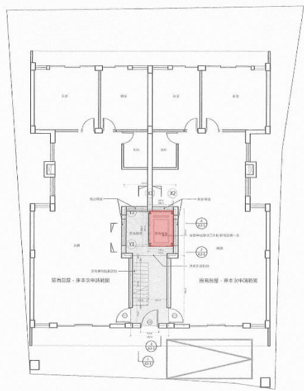
1 A2-1 壹層平面圖 Scale 1/100
